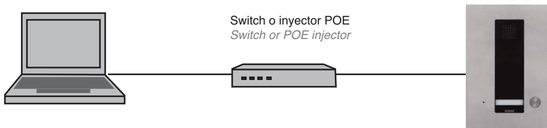
Conexión a un PC a través de elementos POE
